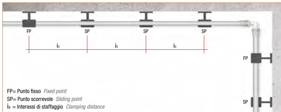
Schema staffaggio a punto fisso FP + punto scorrevole SP
